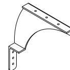
S-2 ×2 ad./pc
