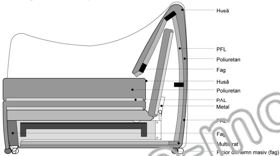
Secțiune canapea extensibilă
