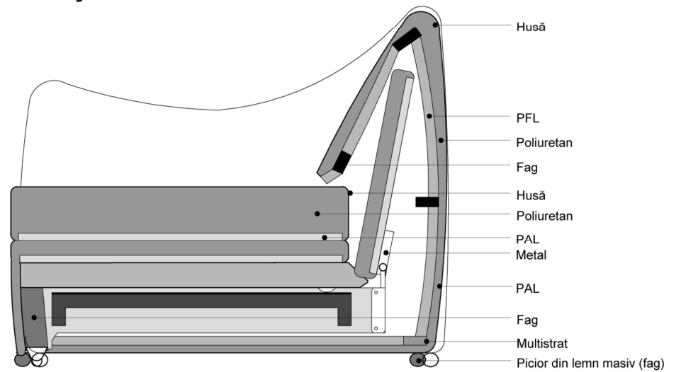
Secțiune fotoliu extensibil
