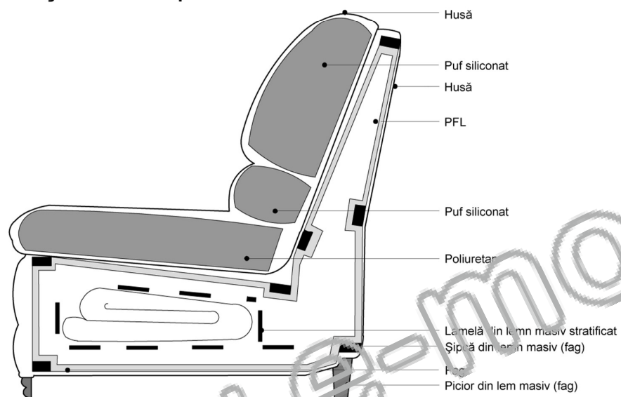
Secțiune canapea extensibilă
