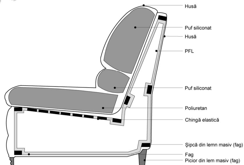
Secțiune canapea fixă
