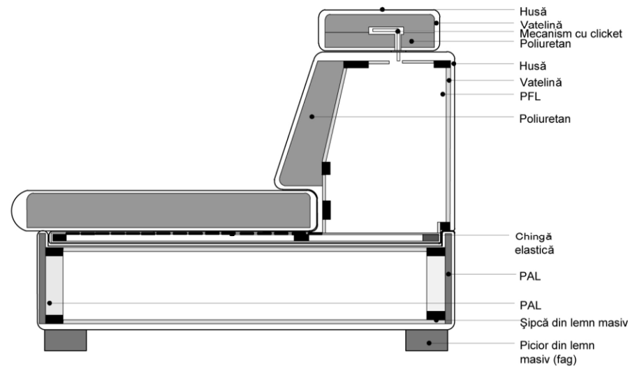
Secțiune ladă fixă
