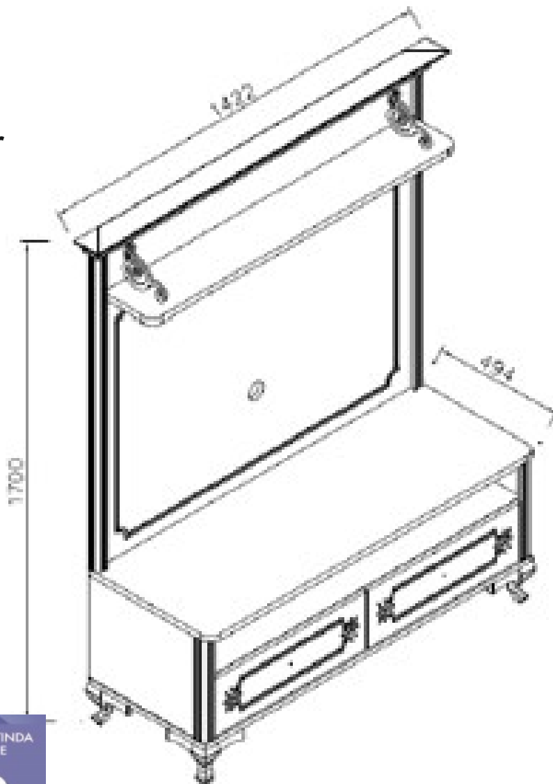
Comoda compacta pt. televizor
